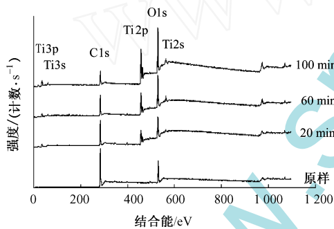
图 4 样品 XPS 全谱扫描图 Fig. 4 XPS survey spectra of samples
