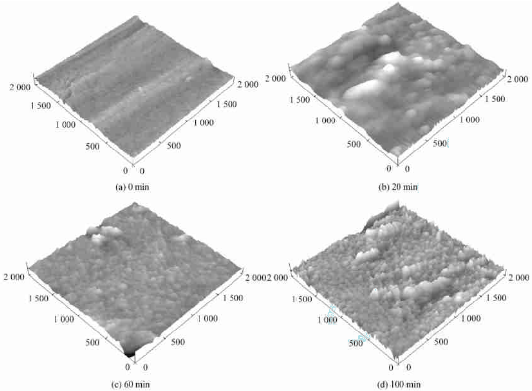
图 1 不同溅射时间制备的 PET 基 TiO 2 薄膜表面 AFM 形貌 (2 000 nm × 2 000 nm)
